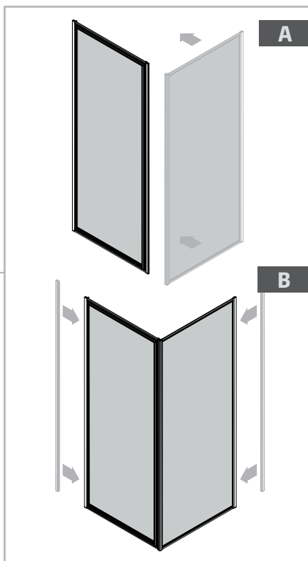
Fig. 2C Position cadre de la cabine
